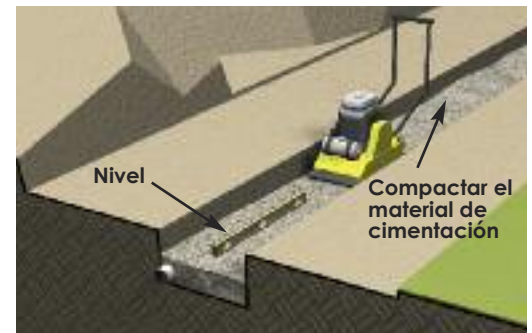
Instalación y compactación del material de cimentación.
