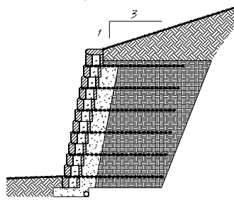
Talud Superior
