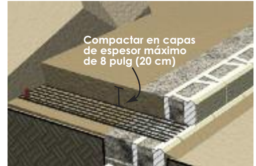
Compactar en capas de espesor máximo de 8 pulg (20 cm).
