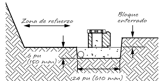
Sección Transversal del Replanteo de la Hilada Base de un Muro Reforzado
