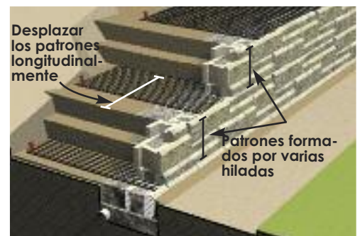
Instalar la geomalla y los patrones siguientes.
